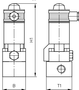
Клапан с соединительным блоком
